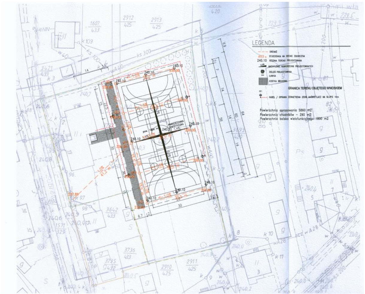
Budowa wielofunkcyjnego boiska sportowego ogólnie dostępnego dla dzieci i młodzieży przy Szkole Podstawowej im. Józefa Kassolika przy ul. Żubrów 13; Mapa zasadnicza, skala 1:1000
